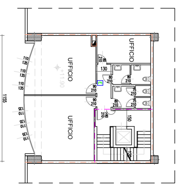
PIANTA PIANO PRIMO ZONA UFFICI
