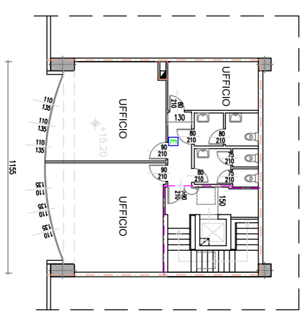
PIANTA PIANO SECONDO ZONA UFFICI
